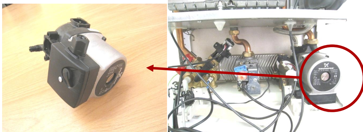
پمپ سیرکولاسیون
